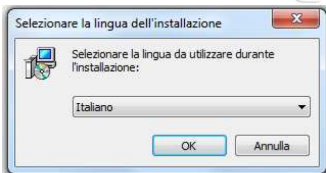
Figura 5: Lingua dell'installazione
